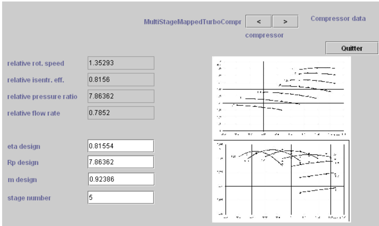
Figure A.8 : Ecran de dimensionnement d'un turbocompresseur avec cartographie
