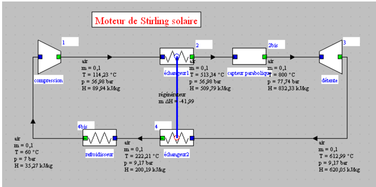
Figure 2.1 : Moteur Stirling solaire
