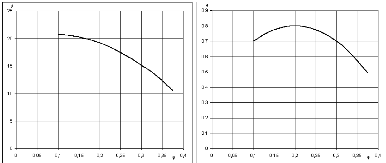
Figure 3.3 Caractéristiques réduites simplifiées d'un turbocompresseur
