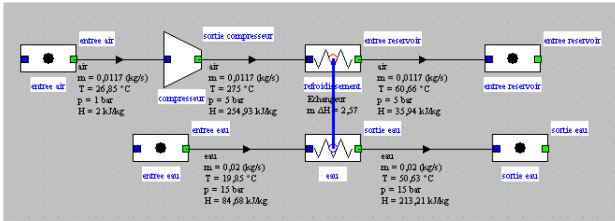
Figure 4.1 : Exemple de compresseur refroidi
