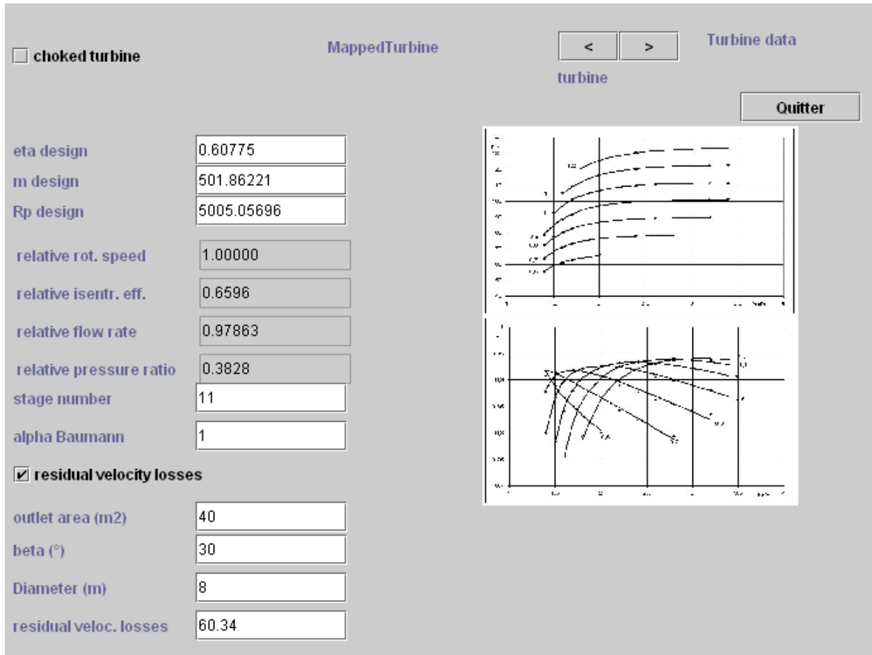
Figure A.4 : Ecran de dimensionnement d'une turbine avec cartographie
